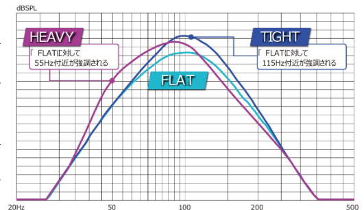
<周波数特性>
